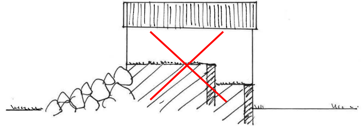
Schéma type d'une construction sur butte avec enrochement et soutènement : interdit
